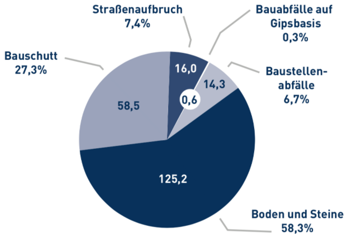
Abbildung 4: Statistisch erfasste mineralische Bauabfälle in Deutschland [Quelle: 11. Monitoringbericht der Kreislaufwirtschaft Bau]
