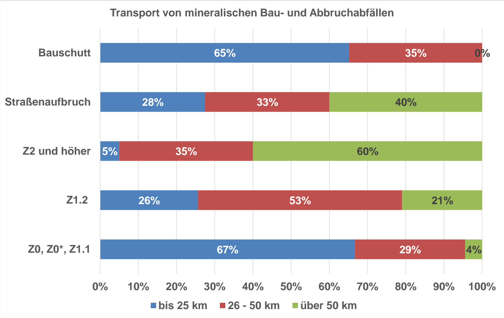
Abbildung 3: Transportentfernungen von Bau- und Abbruchabfällen in Hessen [Quelle: Ergebnis der Umfrage der Mitgliederbefragung des VbU Hessen im Sommer 2018]
